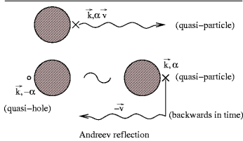
Fig.7. Andreev Reflection
